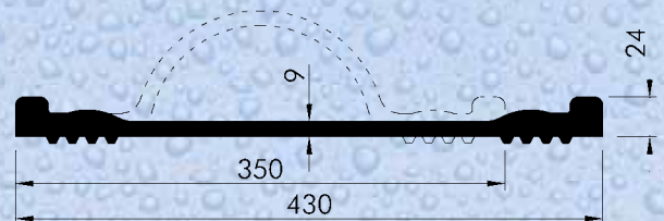
OKB 35 flach mit Gewebe / OKB 35 flat with incorporated textile Elastoflex® nach DIN 7865, Teil 2 / Elastoflex® to DIN 7865, part 2
