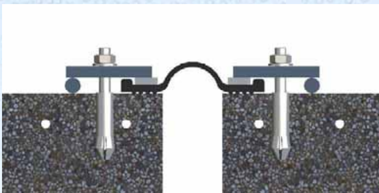
Beispiel: Aufbau einer Klemmkonstruktion mit Kippflansch / Example: mounting of clamped construction with canted flanges
