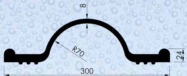
OKB 30 mit Gewebe / OKB 30 with incorporated textile Elastoflex® nach DIN 7865, Teil 2 Elastoflex® to DIN 7865, part 2
