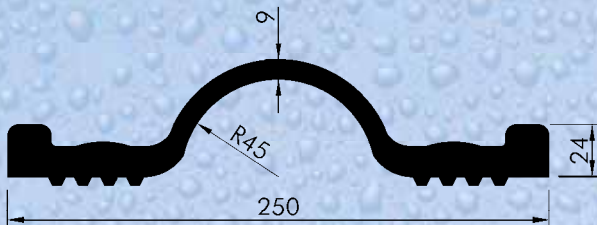
OK 25 Elastoflex® nach DIN 7865, Teil 2 Elastoflex® to DIN 7865, part 2
