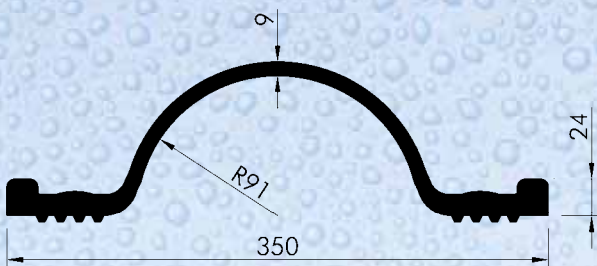
OK 35 Elastoflex® nach DIN 7865, Teil 2 Elastoflex® to DIN 7865, part 2
