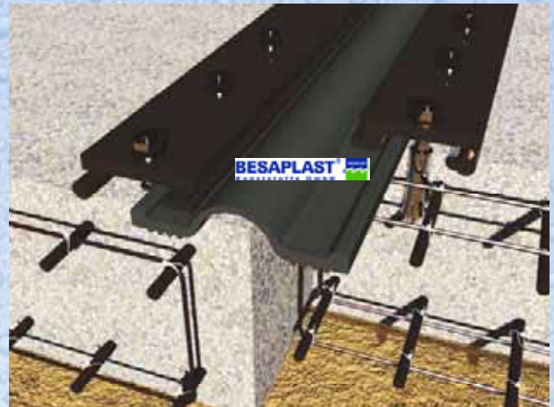
Klemmfugebänder / clamped waterstops
