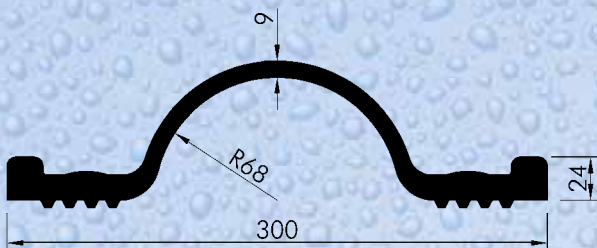
OK 30 Elastoflex® nach DIN 7865, Teil 2 Elastoflex® to DIN 7865, part 2
