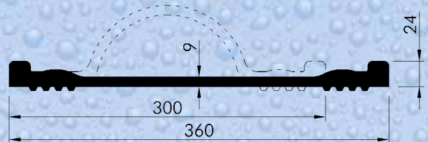
OKB 30 flach mit Gewebe / OKB 30 flat with incorporated textile Elastoflex® nach DIN 7865, Teil 2 / Elastoflex® to DIN 7865, part 2
